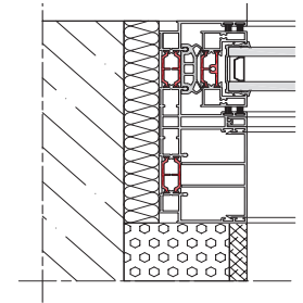
Detail van dorpel bij de configuratie van een verdoken dorpel
