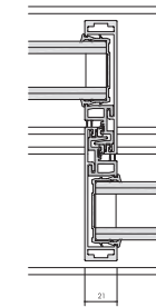
Onderste deel van de configuratie van een vlakke dorpel
