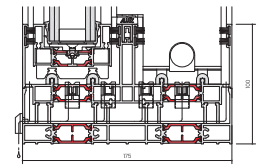
Detail van dorpel bij de configuratie van een verdoken dorpel
